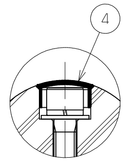
キャップ部詳細 S=1/1
